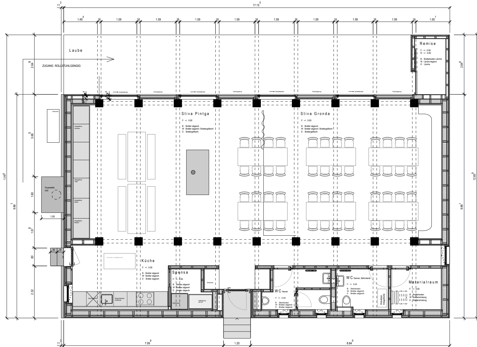
Grundriss Tegia da vout
